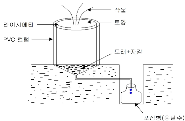
<그림1. 라이시메타 시험도>
